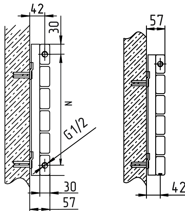
Боковое/Диагональное подключение
